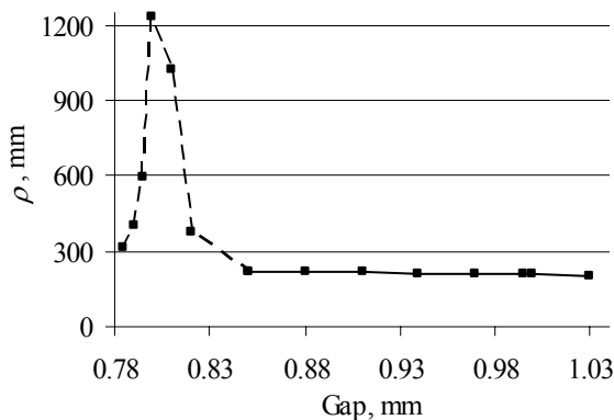
Fig. 14 Radius \rho versus die gap
